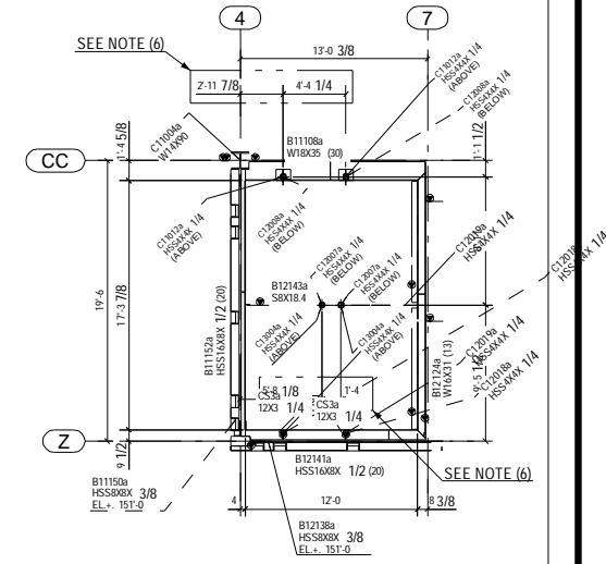
DETAIL A-A
